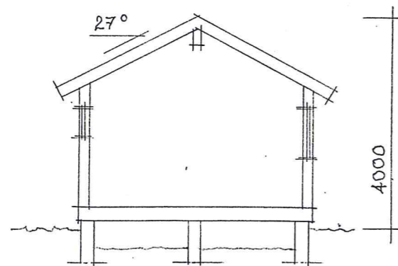
SEKTION A-A
