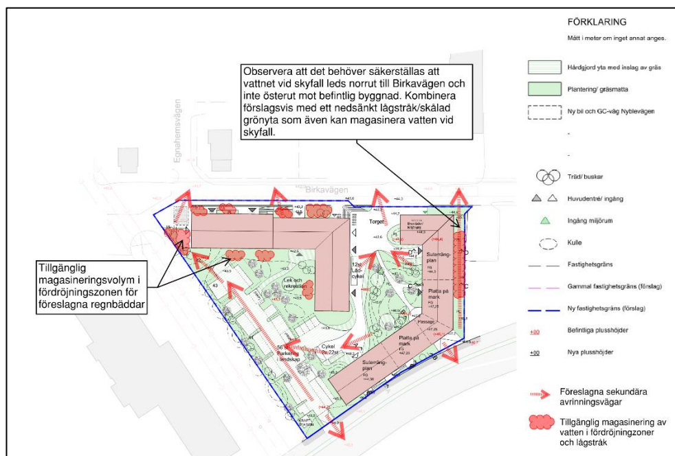
Figur 7:10. Ytliga avrinningsvägar som behöver skapas inom och intill utredningsområdet, samt förslag till möjliga lågstråk/nedsänkta grönytor som kan magasinera ytterligare vatten vid skyfall. Situationsplan tillhandahållen 2025-06-19.
