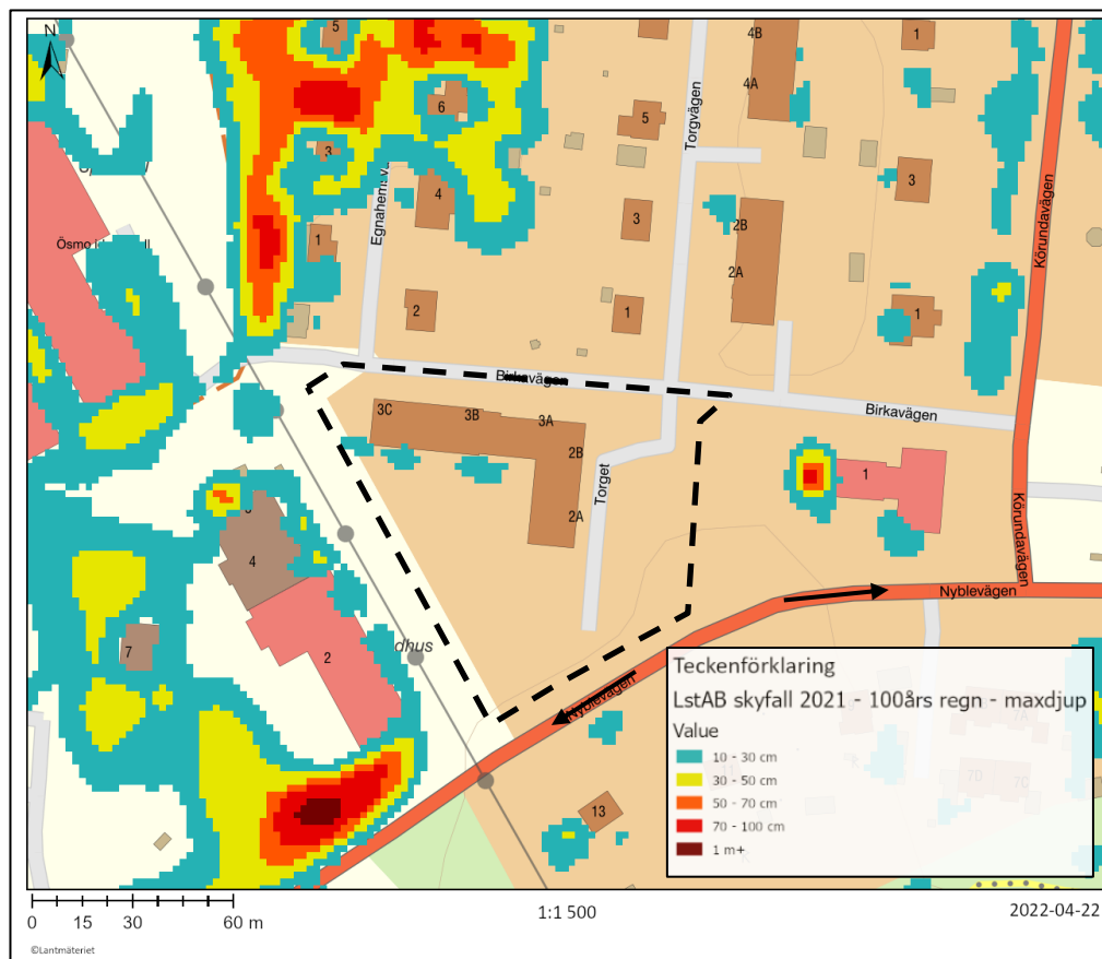
Figur 3:3. Modellerade maximala översvämningdjup vid 100-årsregn inom och intill utredningsområdet, enligt Länsstyrelsens skyfallskartering från 2021. Utredningsområdets ungefärliga gränser är markerade med en svartstreckad polygon.
