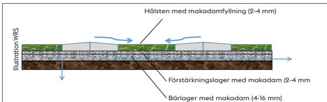
Figur 7:6. Principskiss av en genomsläpplig beläggning i form av gräsarmering, hämtad från Stockholms Vatten och Avfall (2022d).
