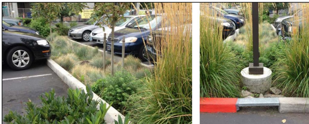
Figur 7:2. Exempelfoto på regnbäddar i gatumiljö där dagvattnet leds in i regnbädden via öppningar i kantstenen (Stockholm Vatten och Avfall, 2022b).
